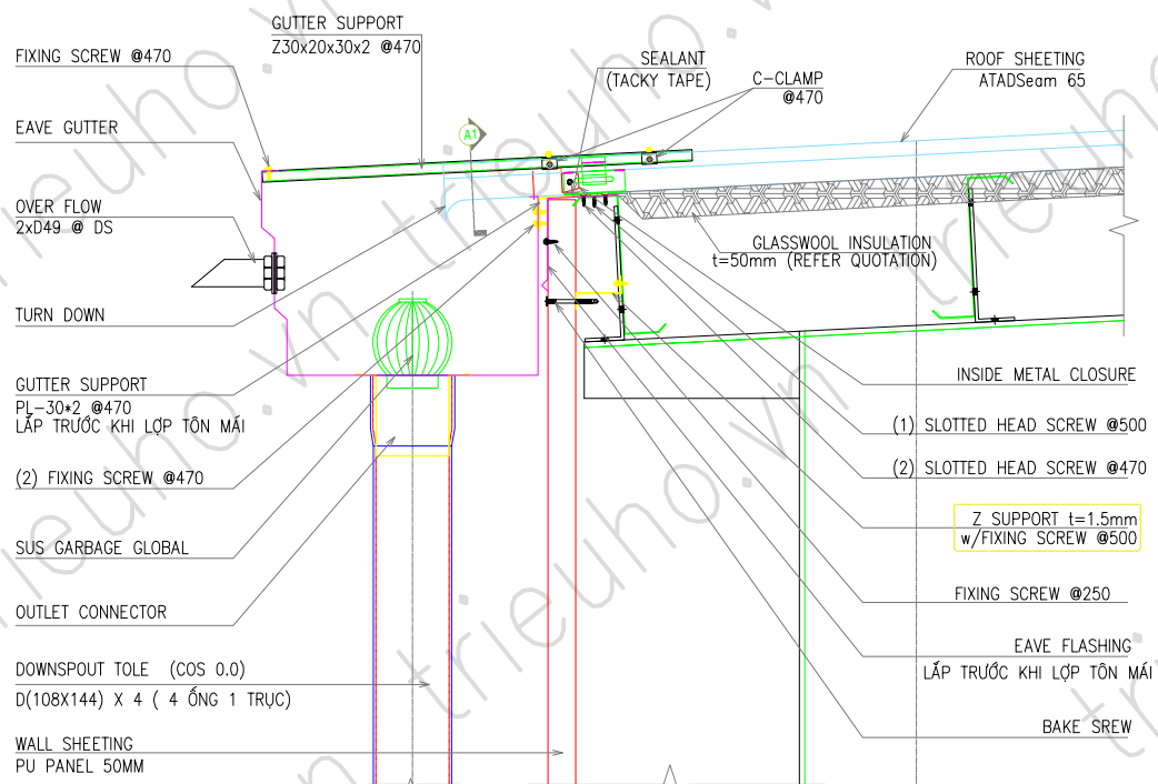
EAVE GUTTER DETAIL (TYP.) @G.L Y1 FRAMING @G.L X1 TO @G.L X17
