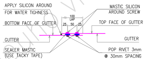
SECTION A2-A2
