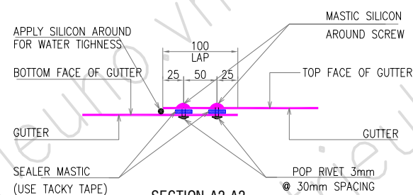
SECTION A2-A2
