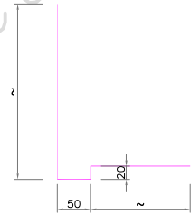
ROLL UP DOOR FLASHING
