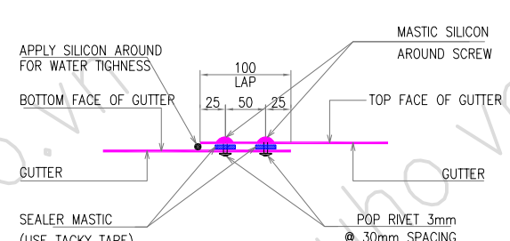
SECTION A2-A2
